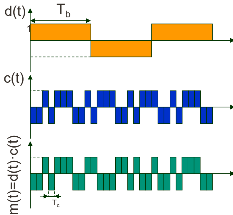
Ensanchamiento (transmisión)
