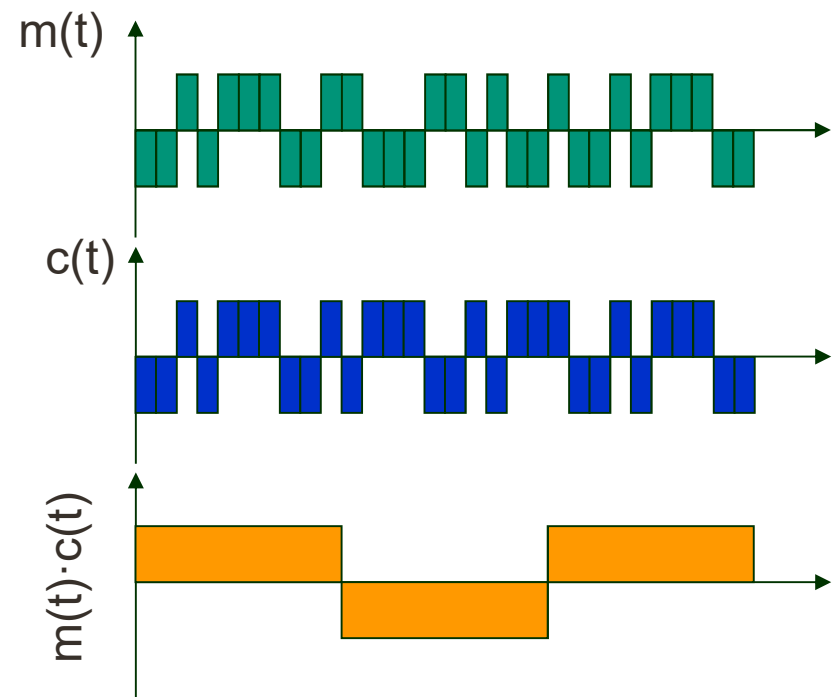
Desensanchamiento (recepción)
