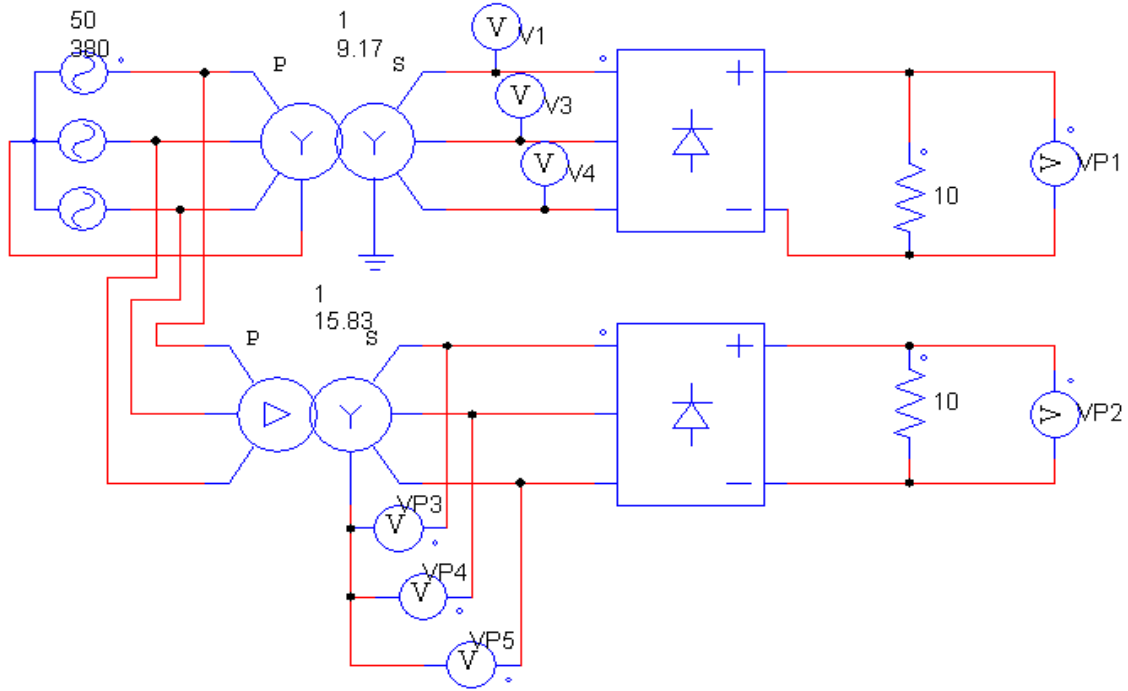
Tensiones de fase y Líneas primario y tensiones fase secundario para el Trafo \Delta -Y con secuencia RTS
