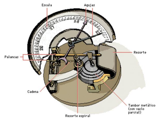
Tubo de Bourdon. Elementos primarios y secundarios en un solo dispositivo
